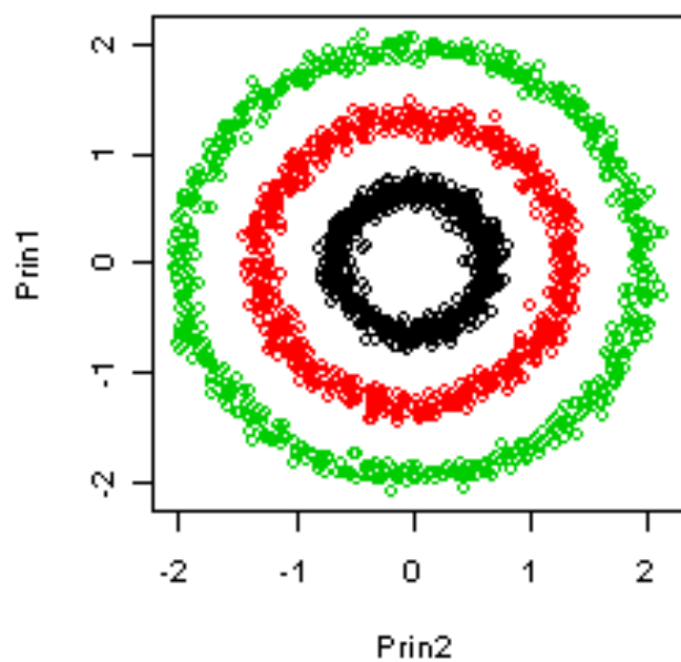
Linear PCA
