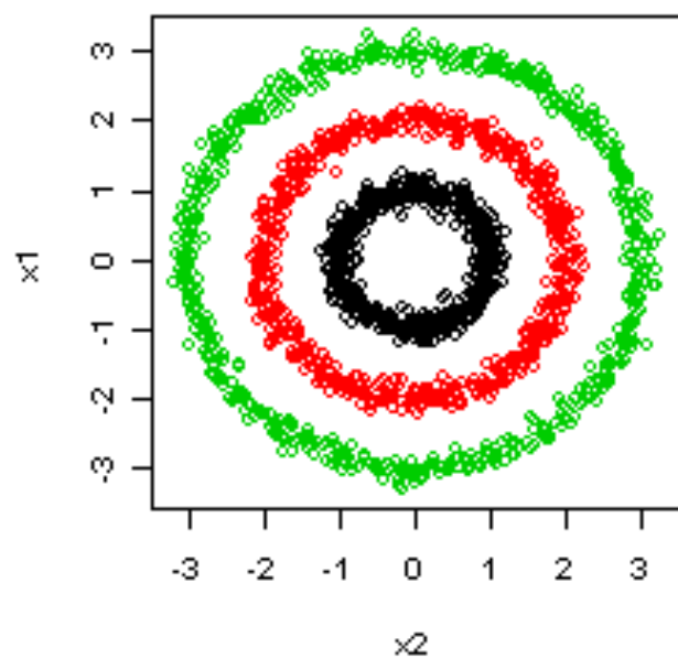
Linear PCA
